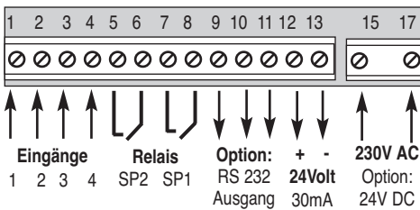
SPE 670 rückseitige Draufsicht
