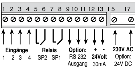
SPE 370 rückseitige Draufsicht
